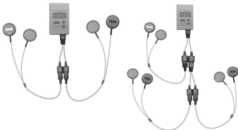
Рис. 5 Подключение виброфонов с помощью разветвителей
